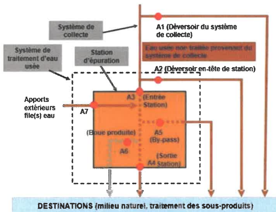
Figure 2 : Illustration schématique de la localisation des différents points réglementaires d'autosurveillance au niveau d'une station de traitement d'eaux usées.
